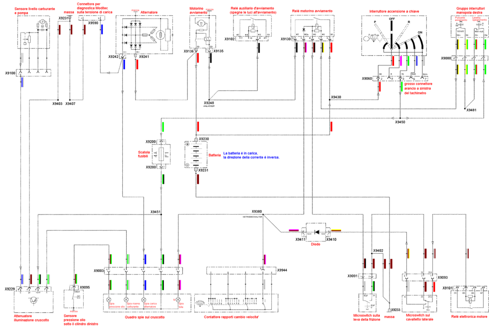
Schema elettrico del circuito di carica e avviamento BMW R1150RT (anche RS)
