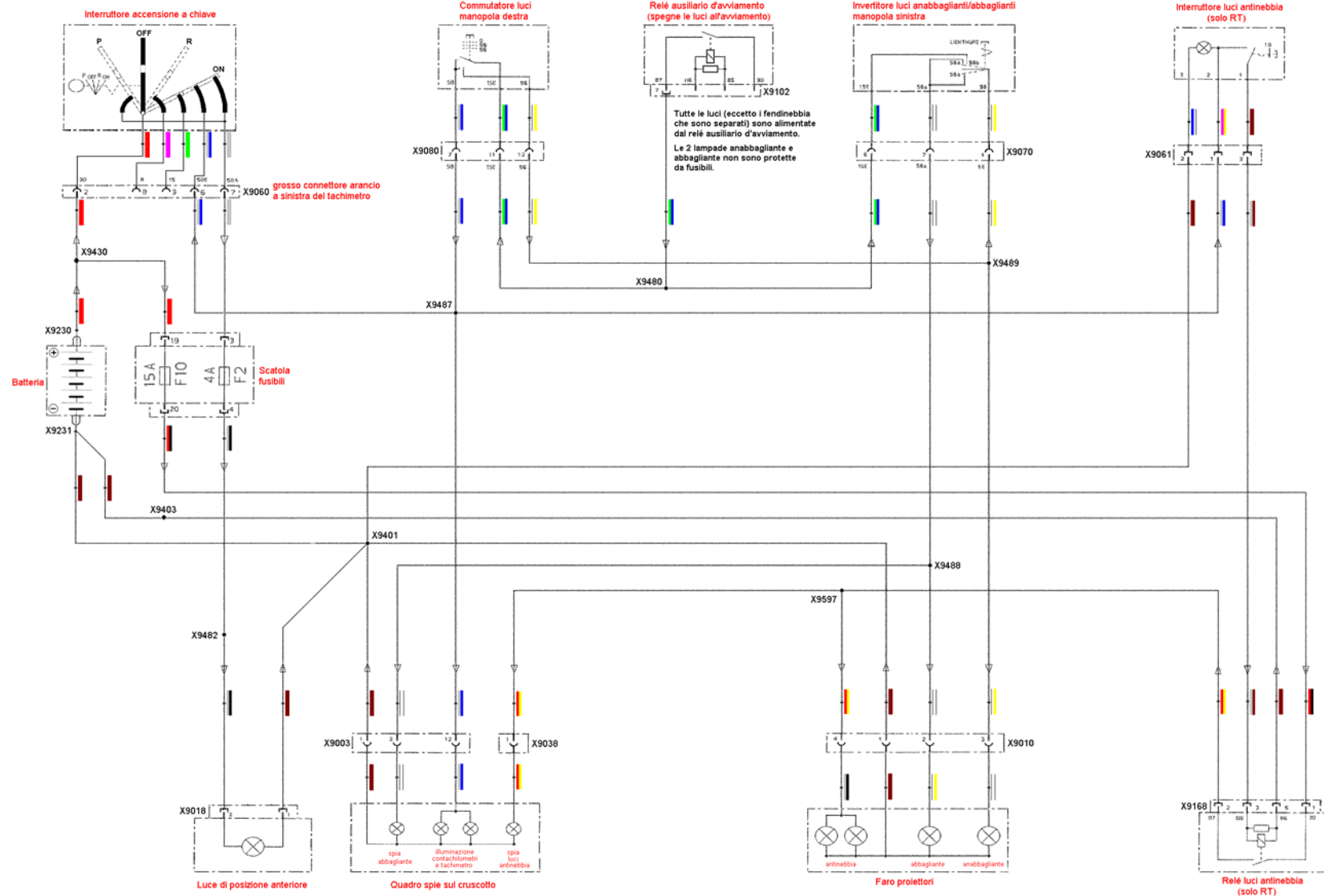
Schema elettrico del Circuito luci BMW R1150RT (anche R-RS-S-GS)
